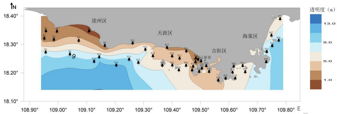
图 2-7 透明度等值线图
