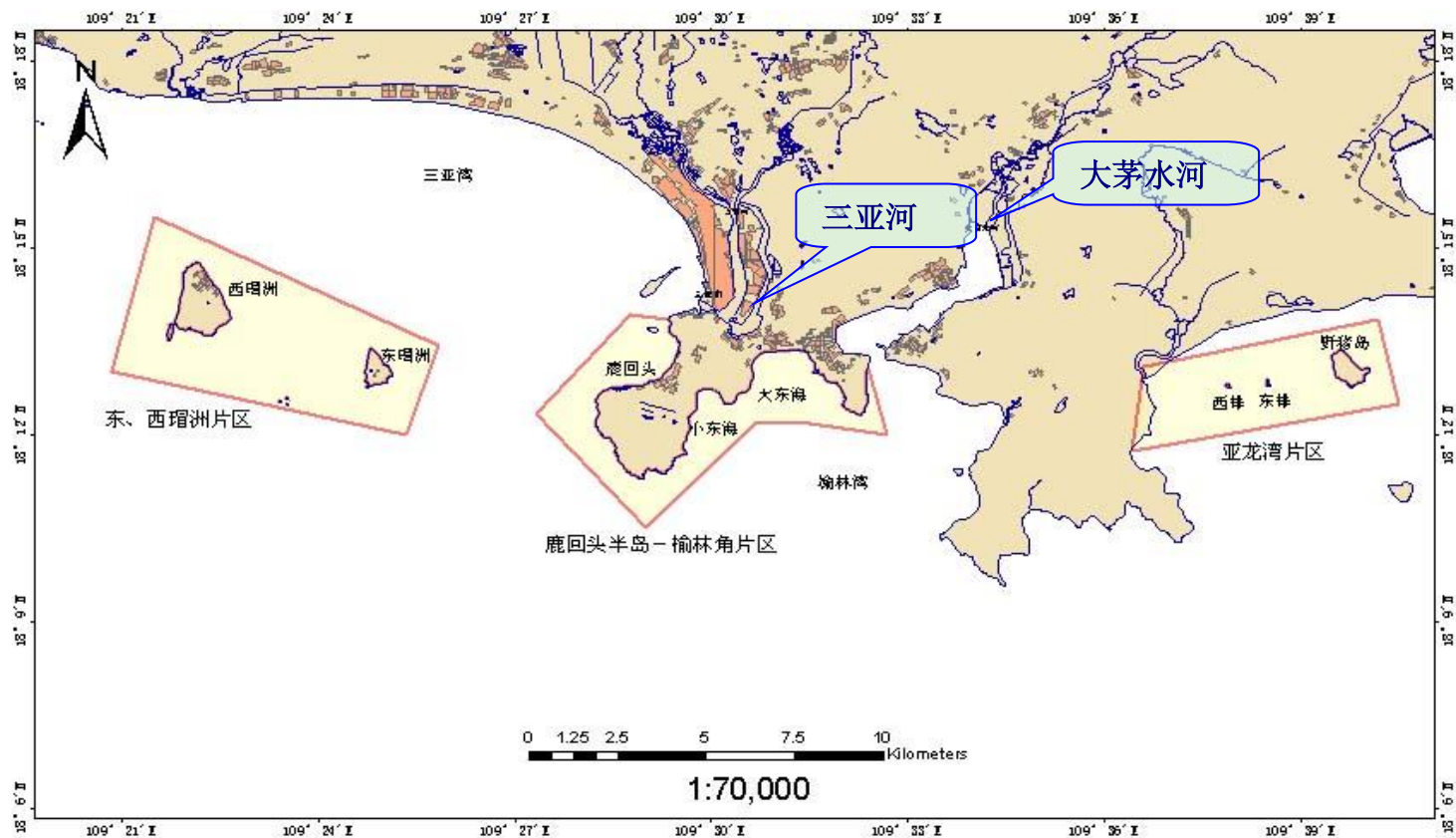
三亚国家级珊瑚礁自然保护区水文地质图
