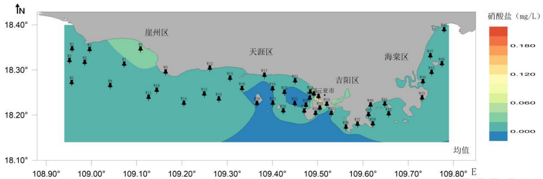
图 2-11 硝酸盐等值线图
