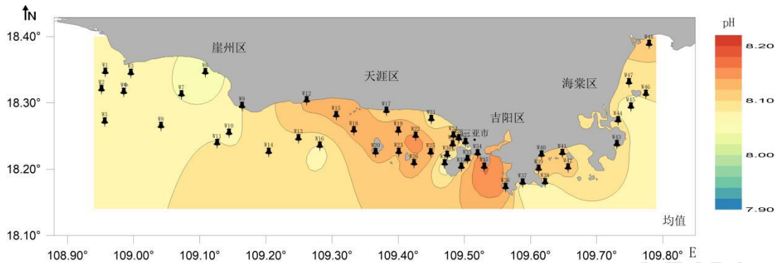
图 2-9 pH 等值线图
