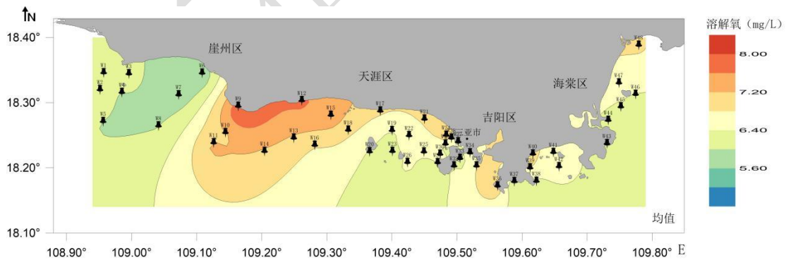
图 2-10 溶解氧等值线图
