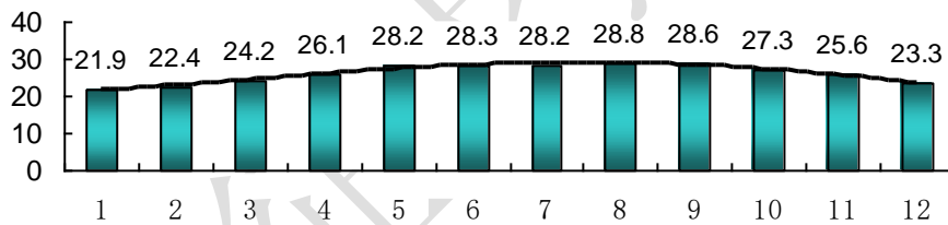
图 2-2 水温各月变化图
