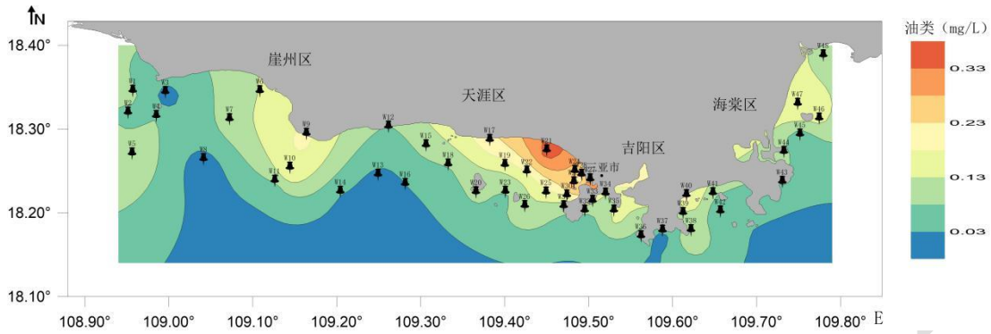
图 2-14 油类等值线图
