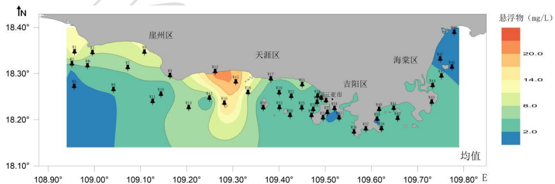
图 2-8 悬浮物等值线图
