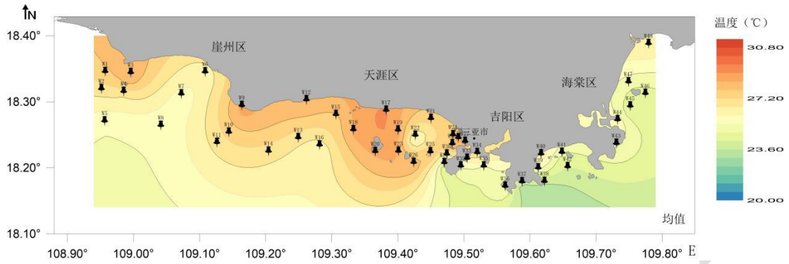
图 2-5 水温等值线图
