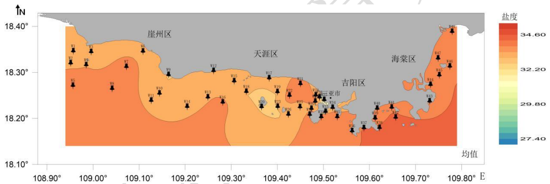
图 2-6 盐度等值线图
