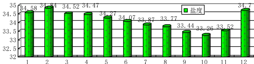
图 2-3 盐度各月变化图
