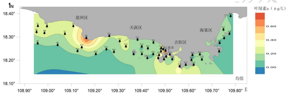
图 2-13 叶绿素 a 等值线图
