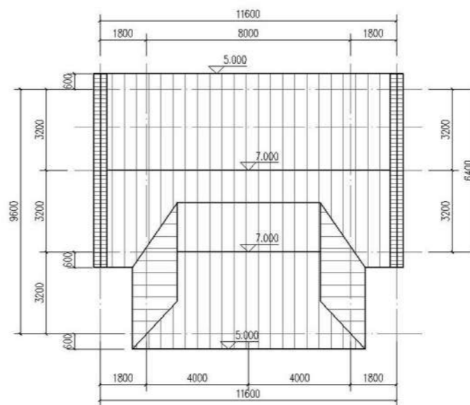
屋顶平面 1:100
